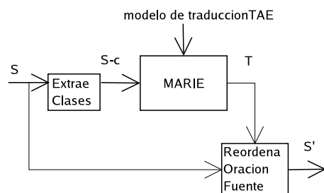
Figura 2: Diagrama de bloques del sistema RAE
